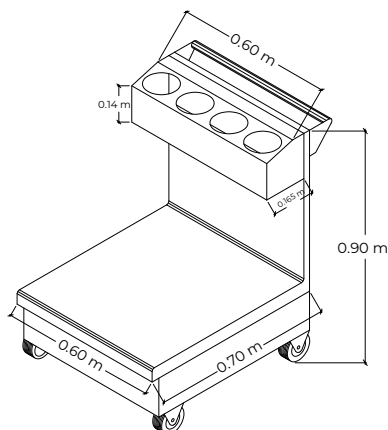
PERSPECTIVA
